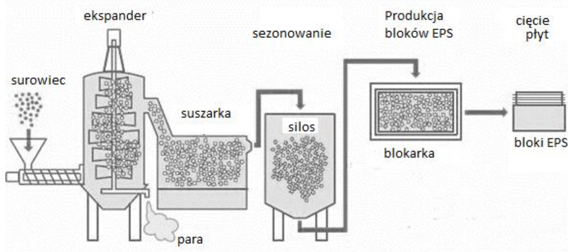
Rysunek 2. Proces produkcji płyt styropianowych
